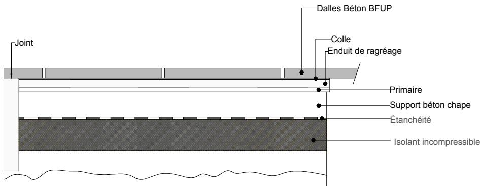
Coupe principe- Fondation Dalles à coller sur sol
